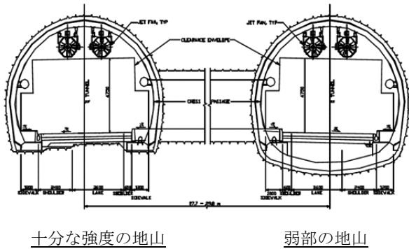
図-4.2 トム・ラントストーンネルの標準断面 (Caltrans hp より)
