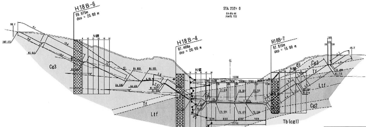
図-9 想定される地質横断面図 (例)
