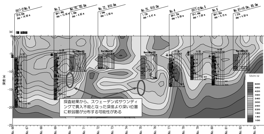
図9 高密度表面波探査結果
