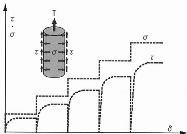
図6 試験の概要
