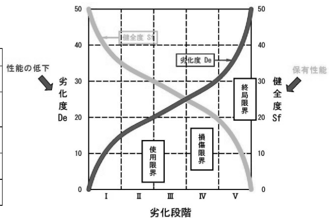
図3 劣化段階および健全度劣化図(表1を図化)
