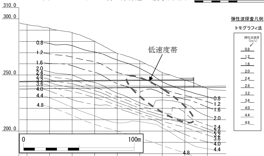
図3 A トンネルの坑口部の弾性波探査結果
