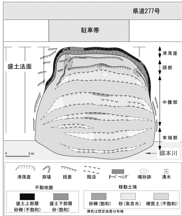
図 3 地質及び変形構造平面図
