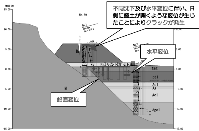
図7 想定される盛土の変状メカニズム
