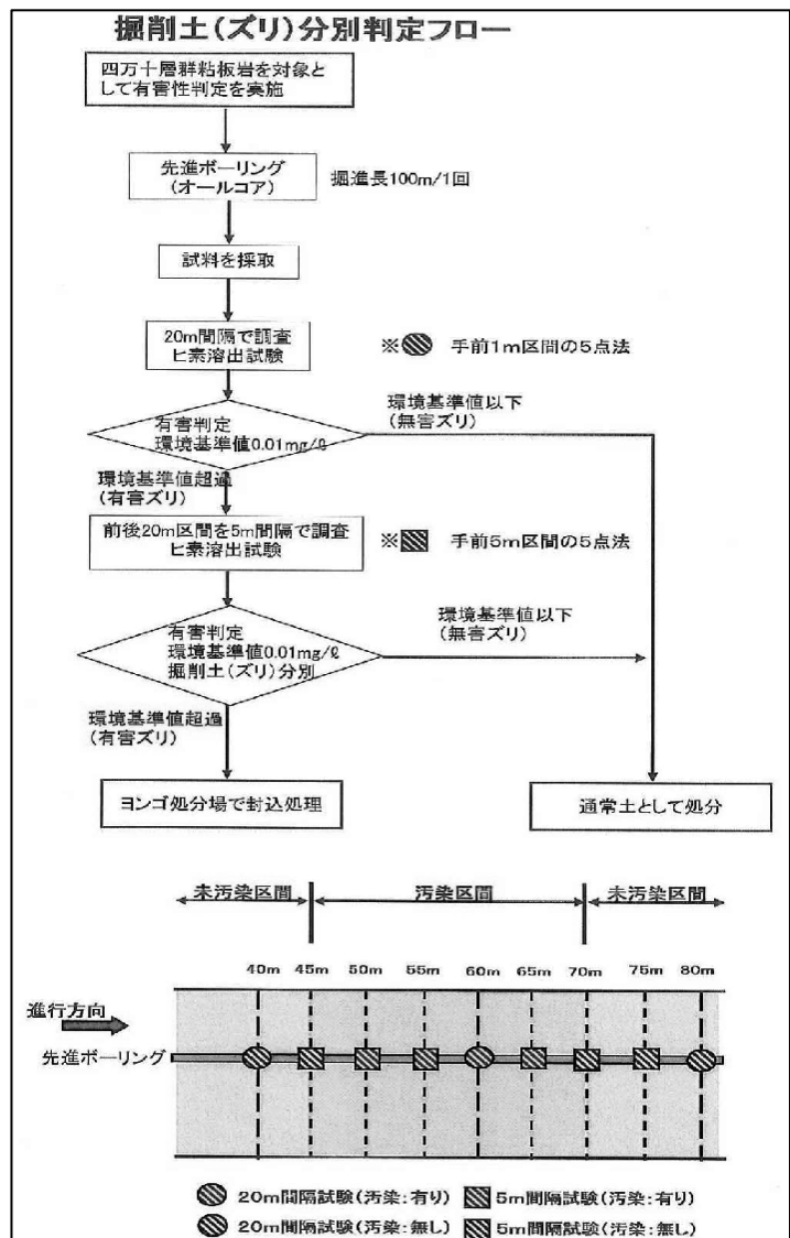
図2 掘削土（ズリ）判定フロー 2)
