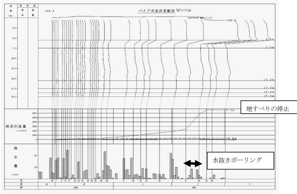
図-4 歪変動図（地すべりブロック内観測孔）
