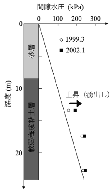
図7 間隙水圧分布(盛土中央直下) 5)
