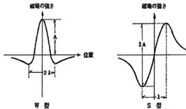
図5 磁気検層測定波形例
