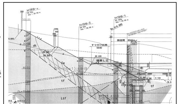
図-3 跨道橋部地質断面図
