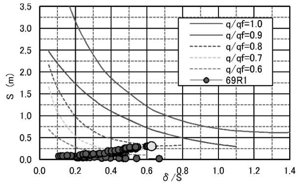
図5 盛土安定管理図 (S~ \delta/S )
