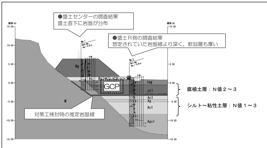
図6 クラック発生箇所の地層横断面図
