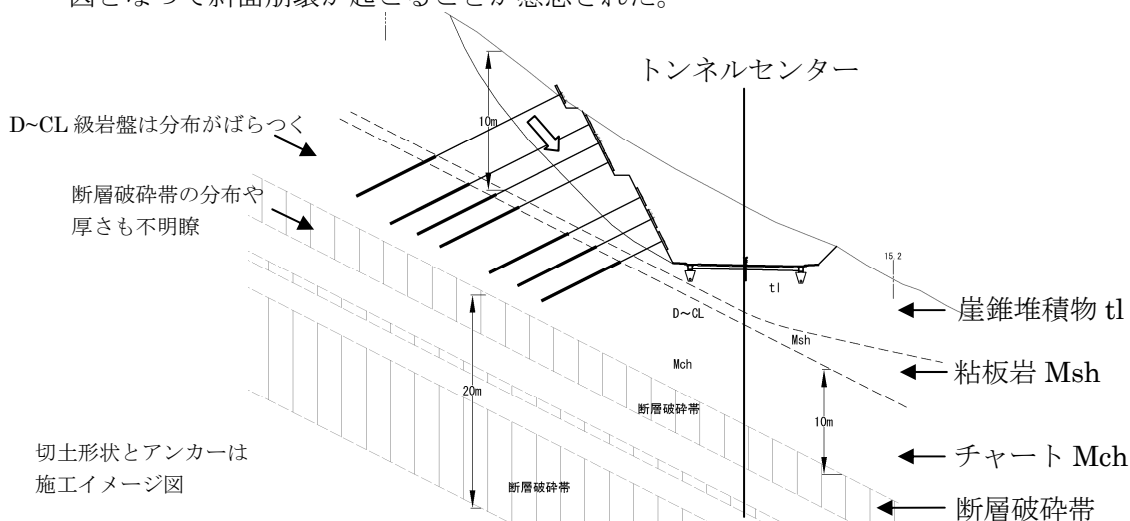
図5 A トンネル坑口部の横断方向の断面図
