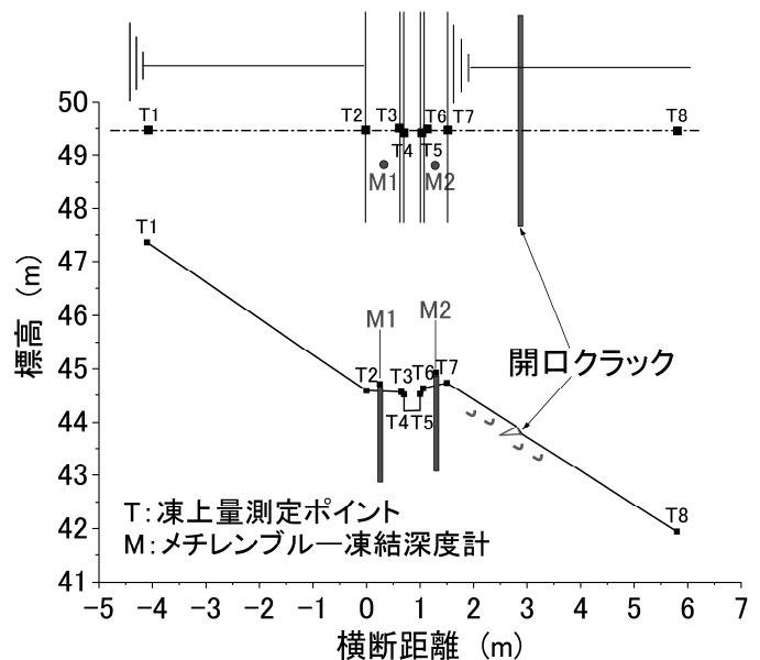
図 2 凍上調査計器配置図
