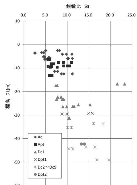
図 5 鋭敏比の深度分布図
