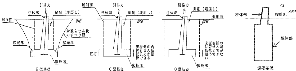
図4 各種基礎形状
