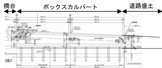
図 2 道路盛土縦断面図
