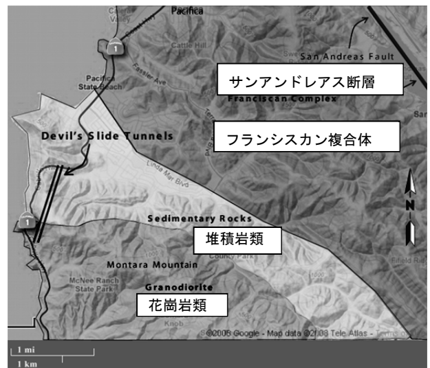
図-4.3 トム・ラントストーンネル周辺の地質平面図 (Caltrans hp より)
