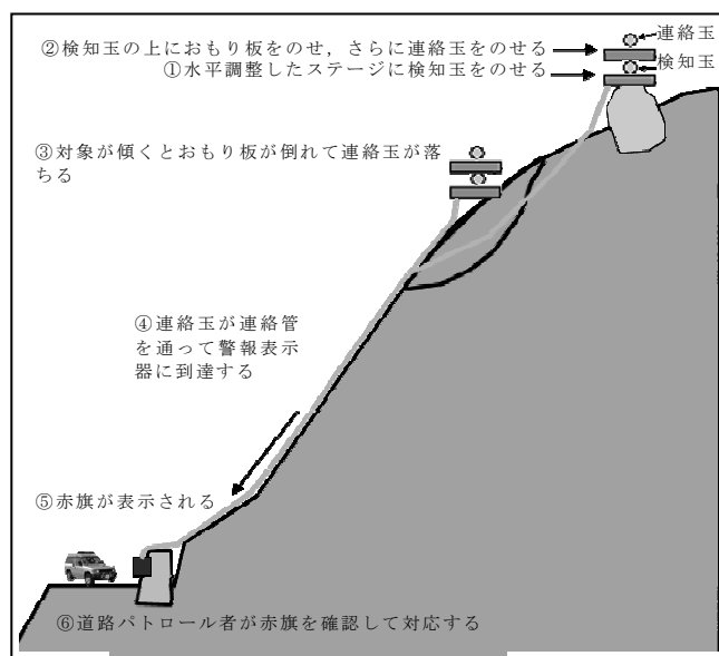
図-1 簡易型傾斜検知器の設置の概要
