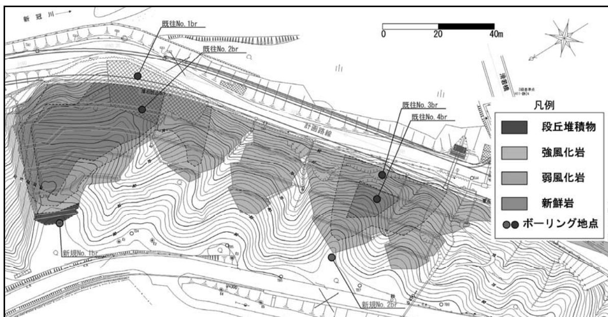
図 1 法面の地質分布
