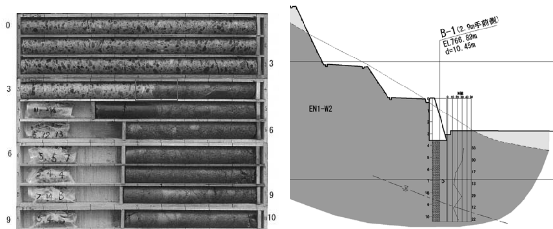
写真 2.2 鉛直ボーリングコア写真 (B-1) と実施位置断面図
