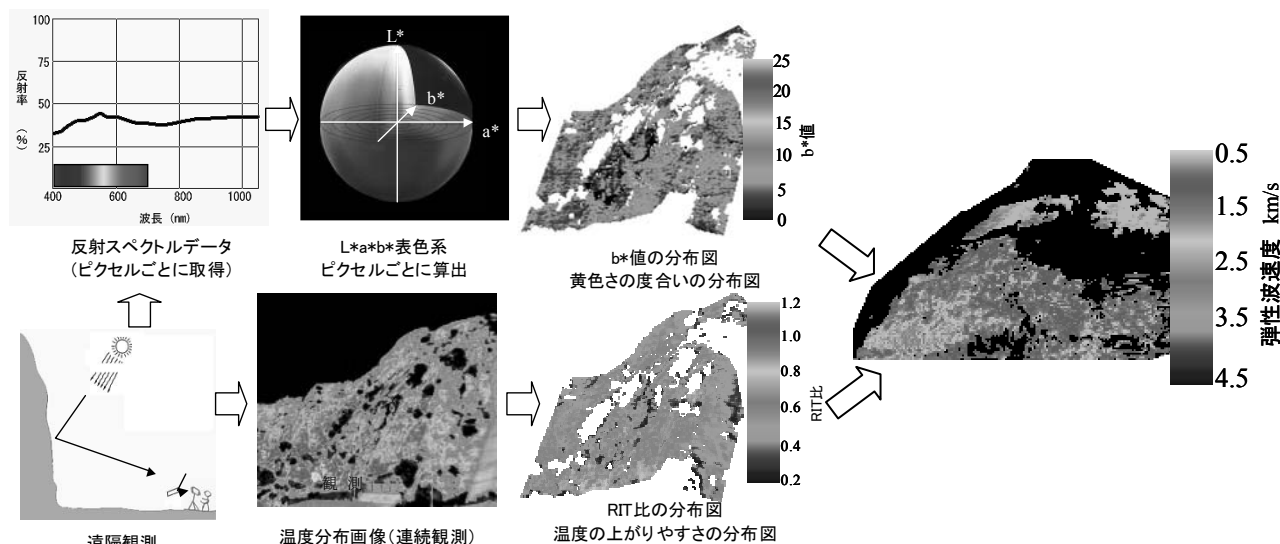
図 10 遠隔観測から弾性波速度推定の流れ
