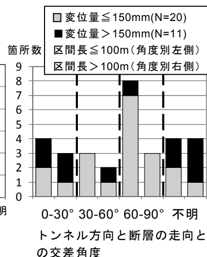
図4 トンネル方向と断層の走向との交差角度の頻度分布
