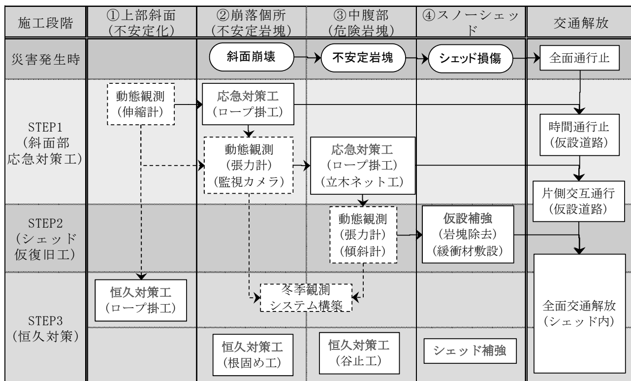
図 2 交通解放までの対策工の流れ
