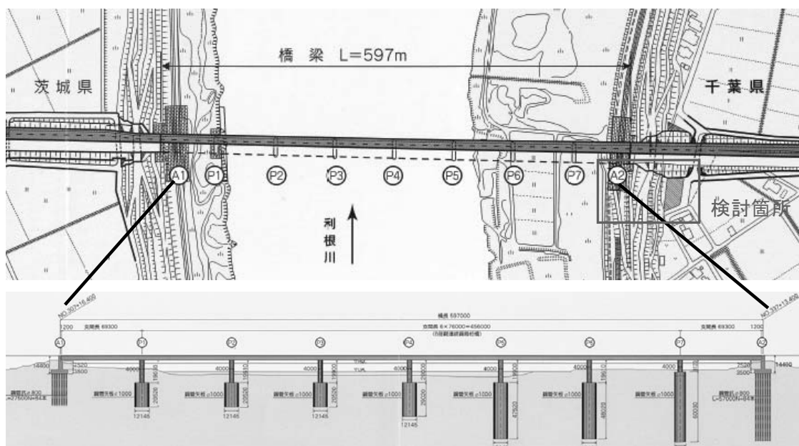
図 3 橋梁部平面・側面図
