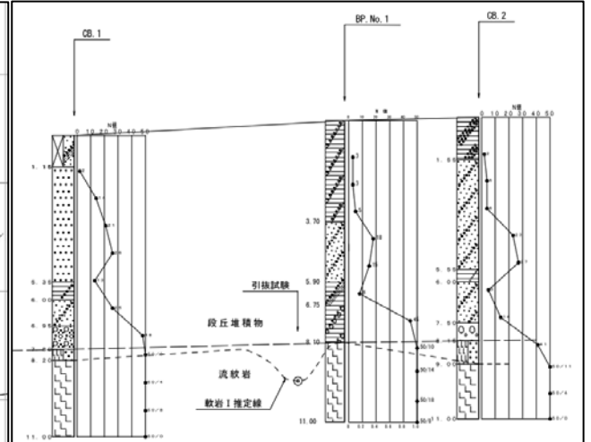
図5 チェックボーリング断面図2
