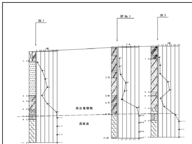
図 3 チェックボーリング断面図
