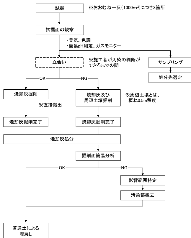
図 3 掘削に掛かる全体のフロー
