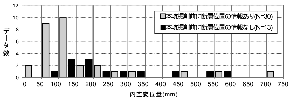
図 1 断層破碎帯における内空変位量頻度分布図
