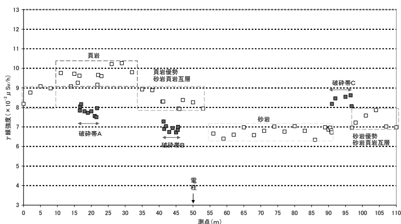
図 5 γ線測定結果図（A 測線）
