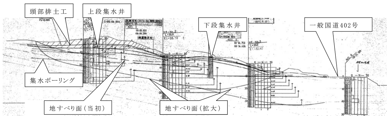
図4 地質断面図(主測線)
