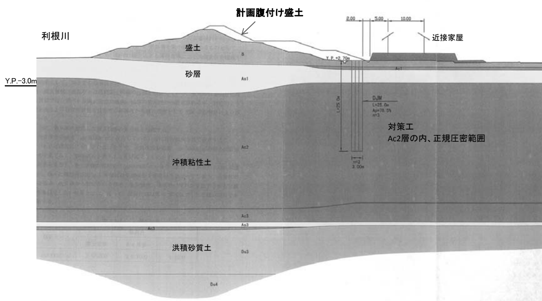
図 4 地盤解析モデルと改良断面図
