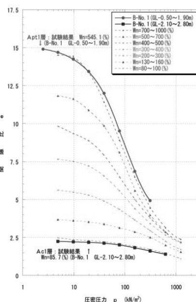
図4 e ~ log p 曲線群
