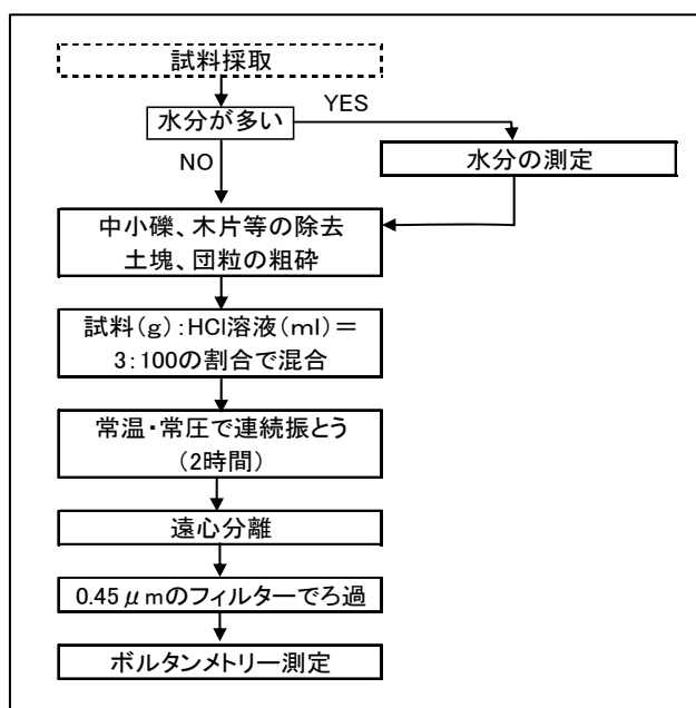
図 5 前処理・分析手順
