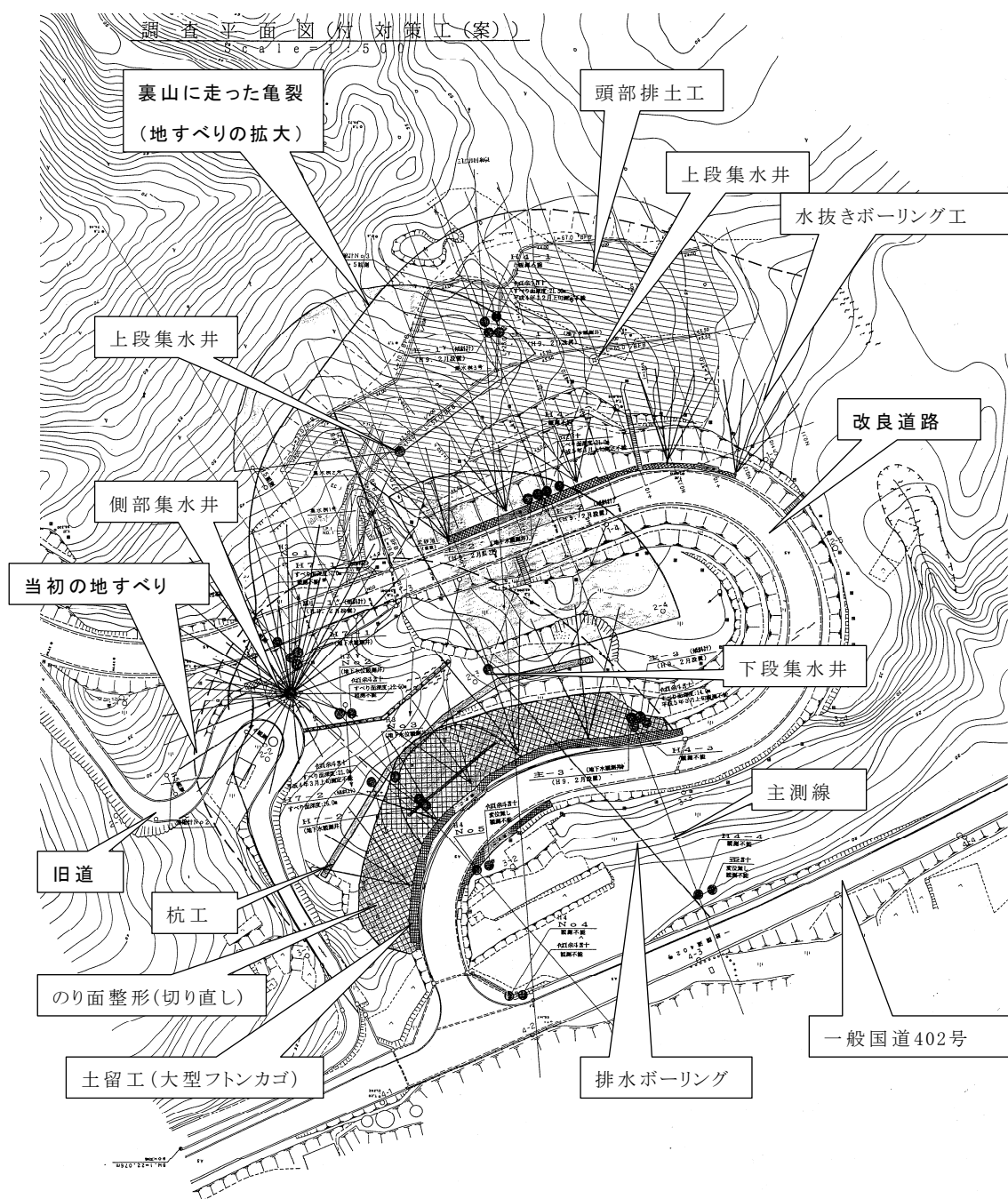
図3 改修範囲平面図(旧道と新道の関係および地すべり対策工の実施状況を示す)
