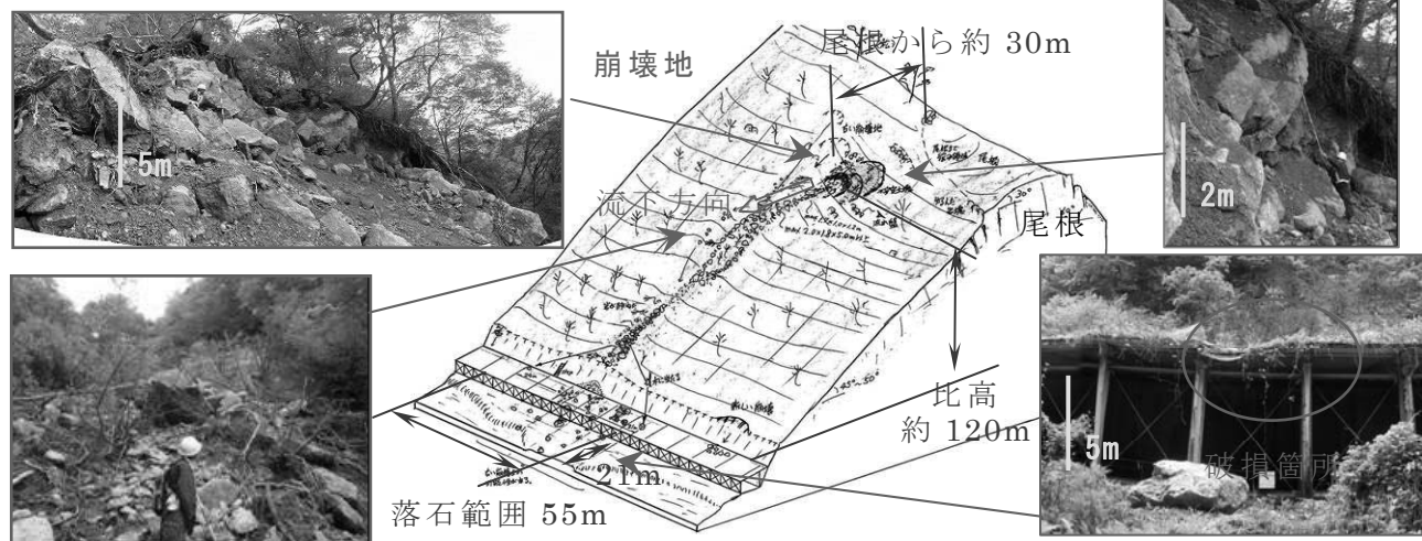
図1 被災状況の概要図
