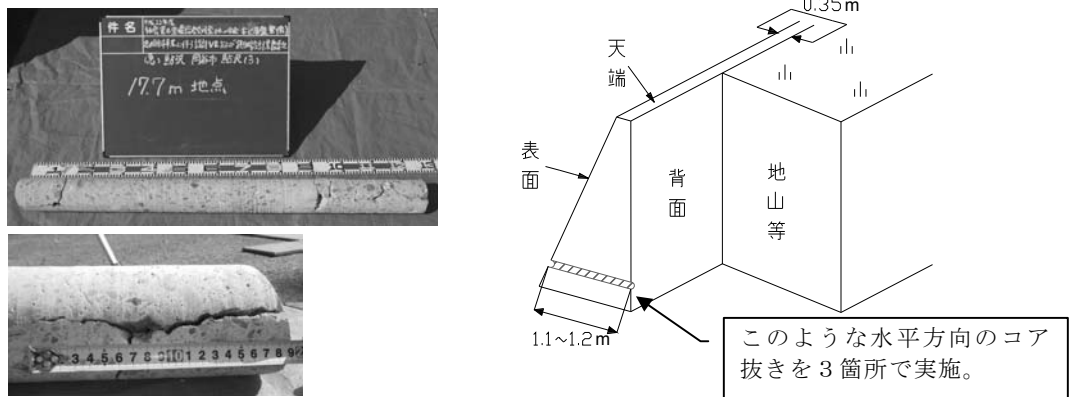
写真 2.1 擁壁の水平コア抜き結果
