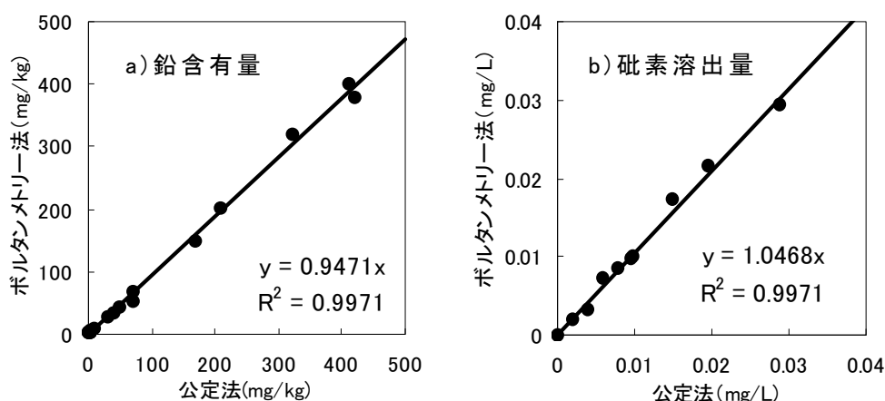
図 6 ボルタンメトリー法と公定法との相関例 [a) 鉛含有量、b) 砒素溶出量]
