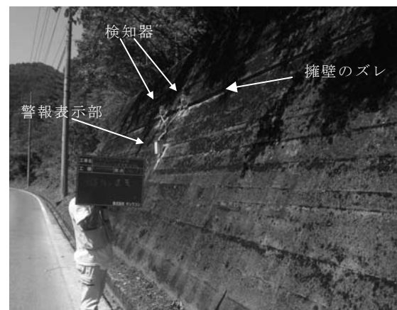
図3 擁壁のズレと傾斜検知器
