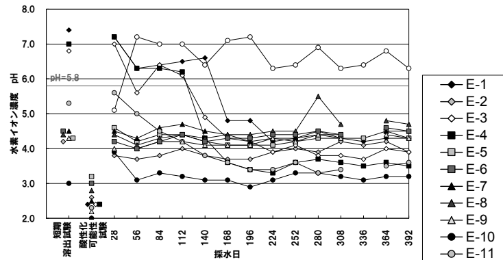
図 3 曝露試験における水素イオン濃度と短期溶出試験の水素イオン濃度の関係
