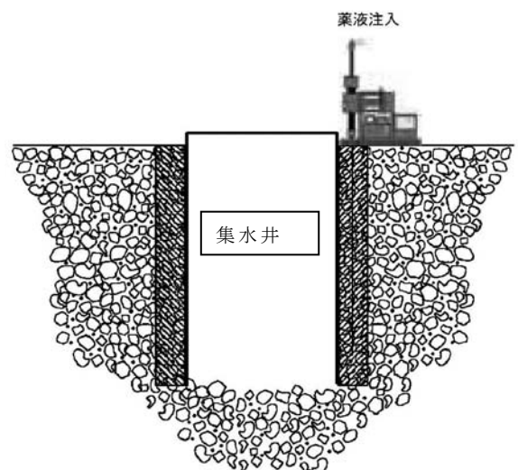
図 3 薬液注入工法イメージ図
