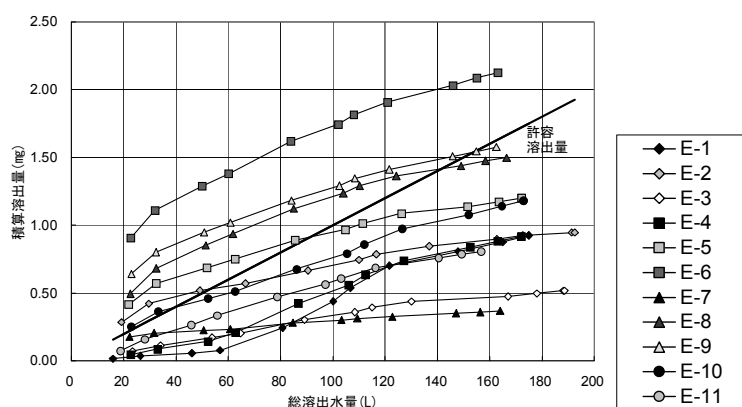
図5 曝露試験におけるセレンの総溶出水量と積算溶出量の関係図
