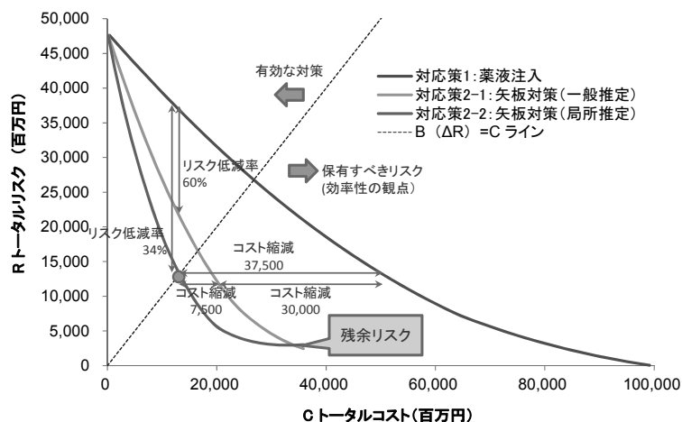
図-9 対策効果と対策投資額の関係
