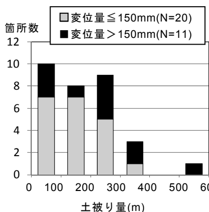
図2 土被り量の頻度分布
