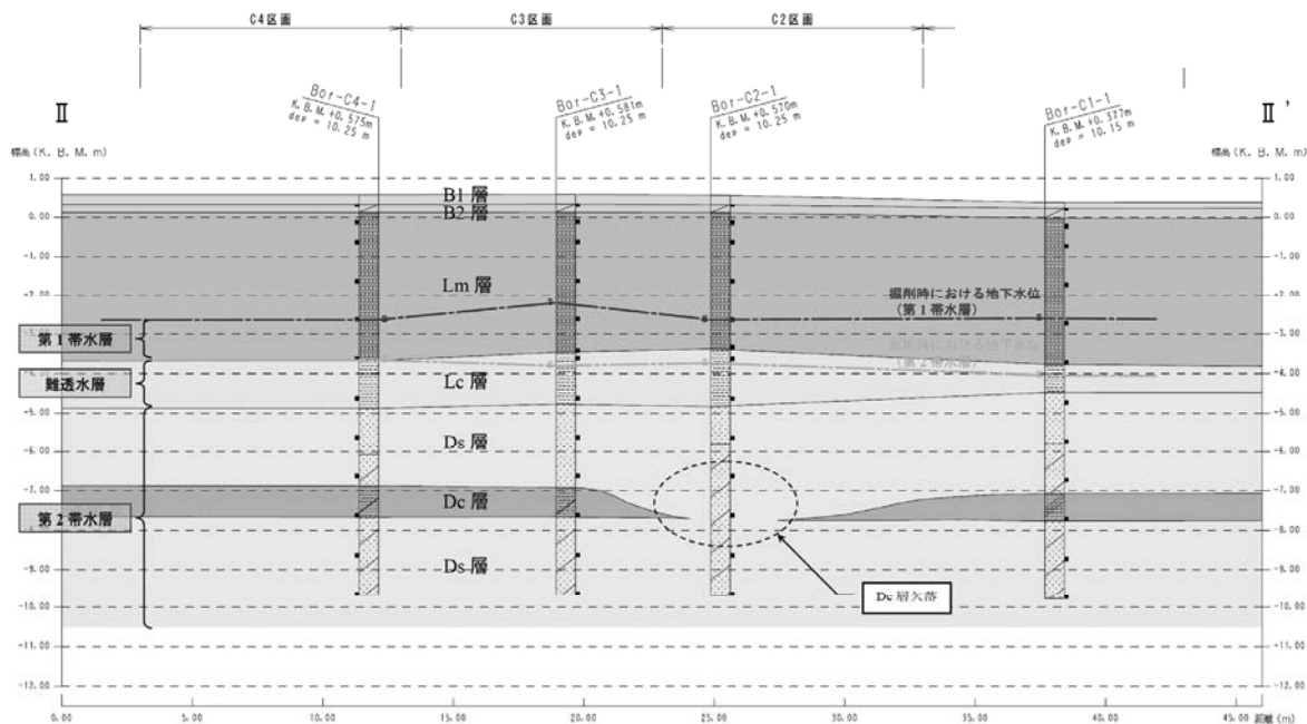
図2 当該地の地質断面図
