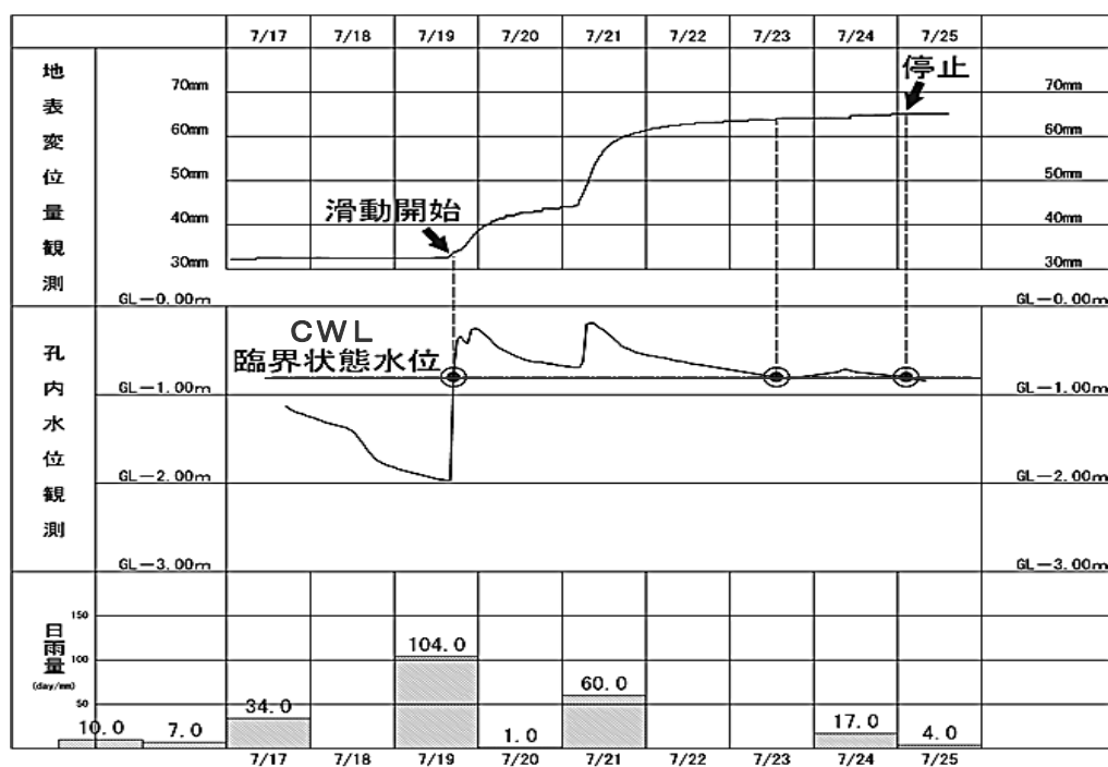
図3 モニタリングによる臨界状態の特定
