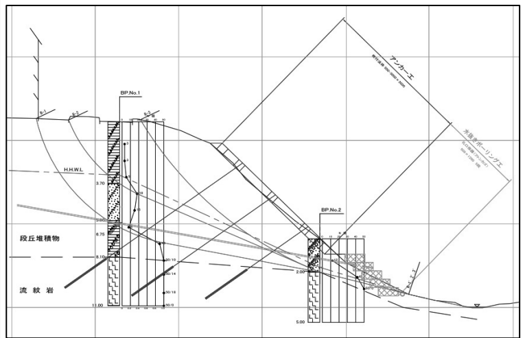
図2 対策工断面図
