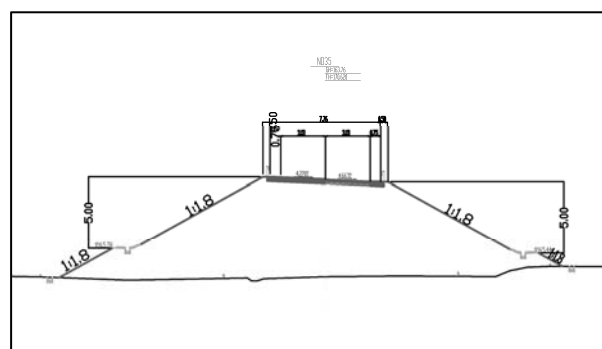
図-2 標準断面
