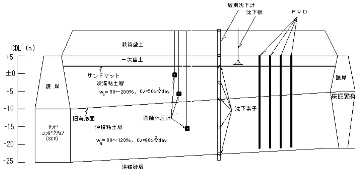
図 2 地盤概要図
