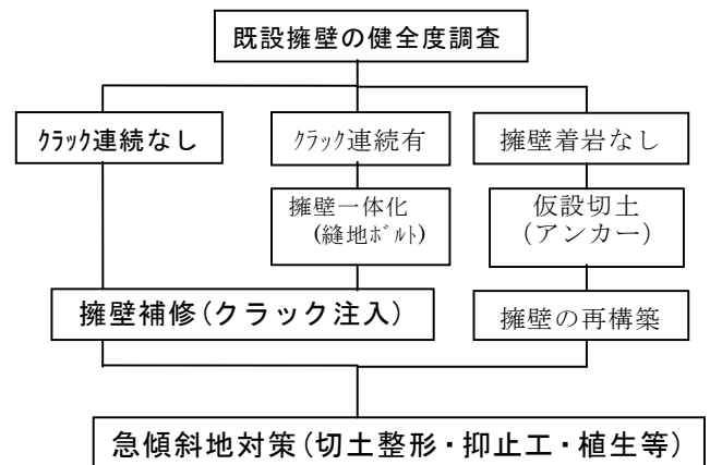
図 2.2 リスク対応方針 2 の場合の検討フロー
