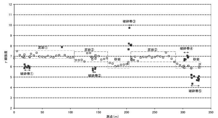
図 7 γ線測定結果図 (B 測線)
