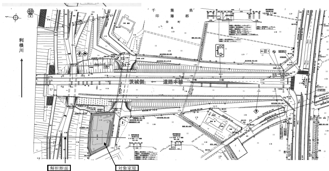
図2 対象地概要図(対象家屋および解析断面位置)
