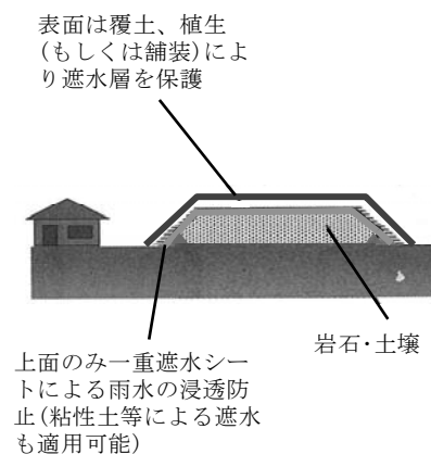
図6 対策工概念図
