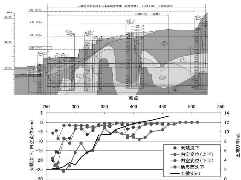
図7 水源工区における地表面沈下・坑内変位
