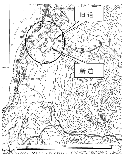
図1 調査地周辺の地形(複数の地すべり様地形が確認できる)
