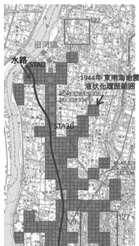
図-2 液状化履歴図（若松 2011 1) に加筆）
