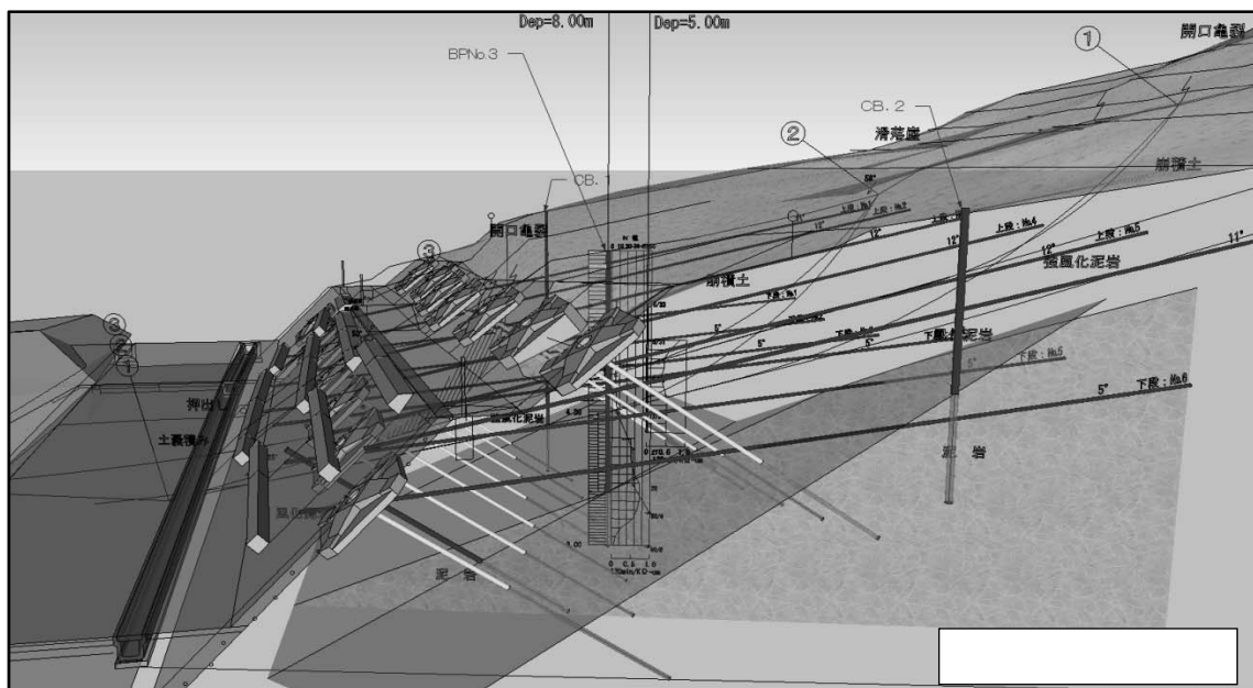
図 1 断面図
