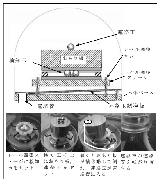
図-2 簡易型傾斜検知器の構造
