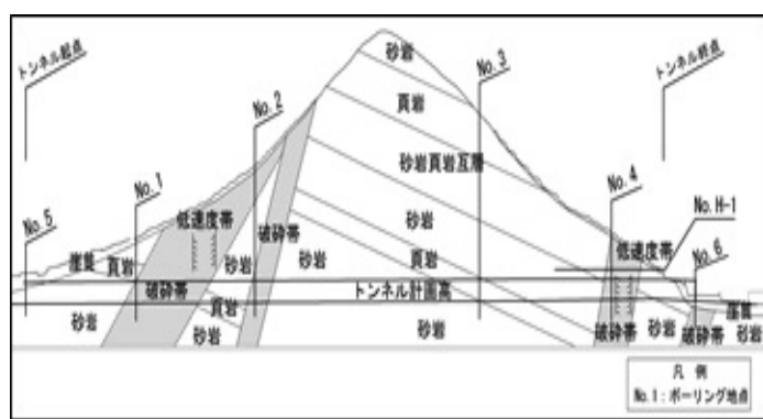
図 4 トンネル地質縦断面図
