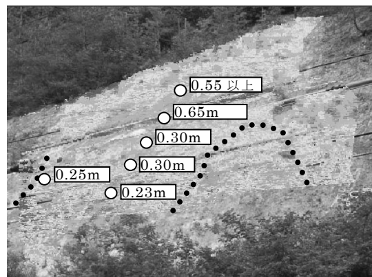
図 13 ドリル削孔による緩み厚さ計測結果
