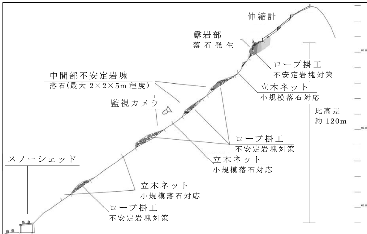
図 4 応急対策工(ロープ掛工・立木ネット：斜面上部から順に施工)
