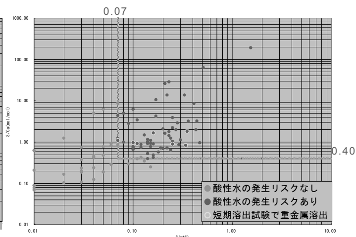
図 2 蛍光 X 線の硫黄含有量 (S) と蛍光 X 線の硫黄含有量の関係図
