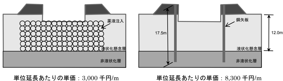
図-4 対策工概要図
