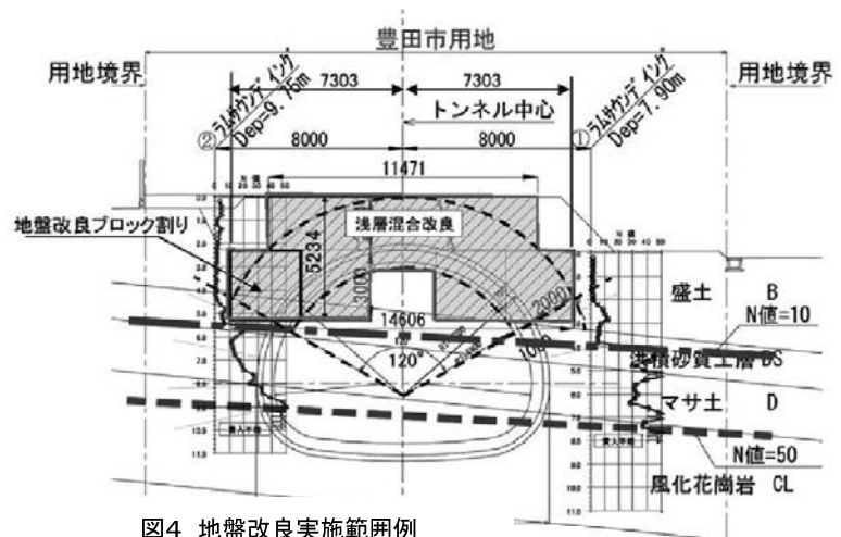
図4 地盤改良実施範囲例
