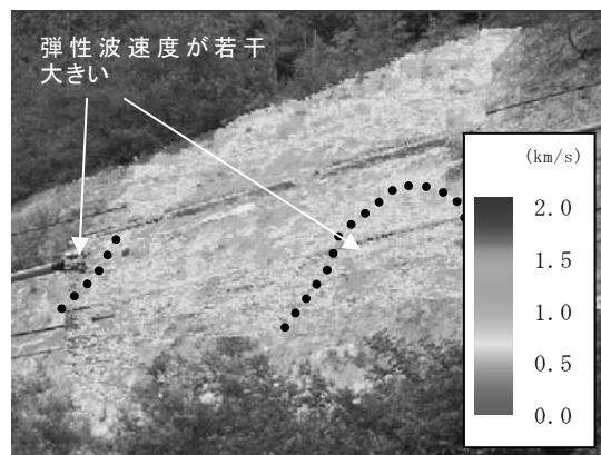
図 12 推定弾性波速度の分布図
