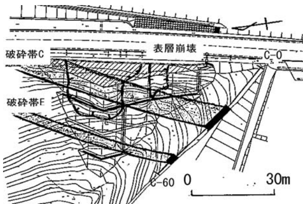
図 8 調査位置図（C 測線）
