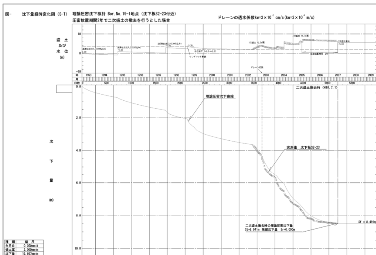
図 4 理論沈下計算と実測沈下の対比状況例
