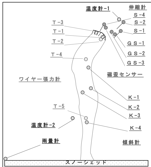
図 5 観測計器位置図
