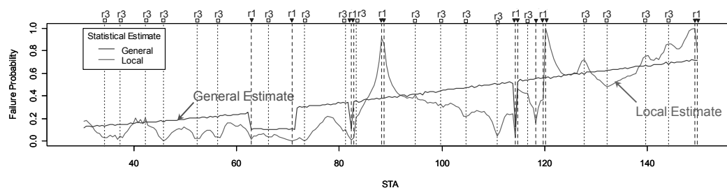
図-8 任意地点におけるリスク事象の発生確率
