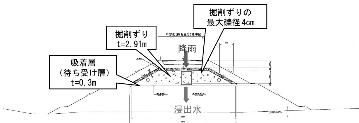
図 1 盛土模式図 (吸着層の場合)
