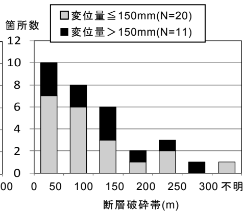
図3 断層破碎帯の区間長の頻度分布
