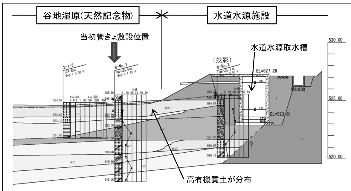
図1 谷地湿原と水道水源施設の断面図
