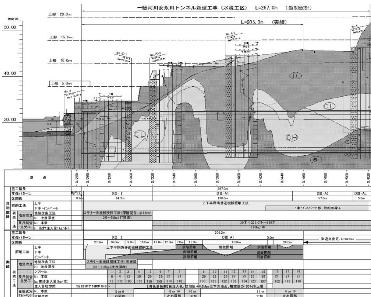
図3 最終確認された地山分布と設計時および施工時の施工内容
