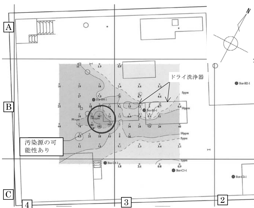
図 4 詳細調査の土壌ガス調査結果（PCE 濃度分布図）
