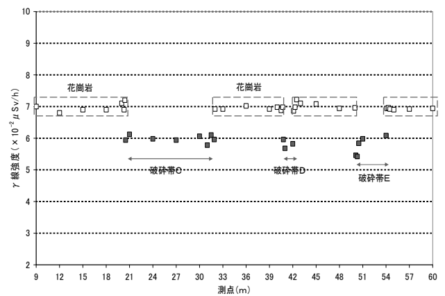
図 9 γ線測定結果図（C 測線）
