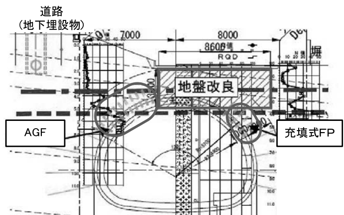
図5 変則的な地盤改良実施例
