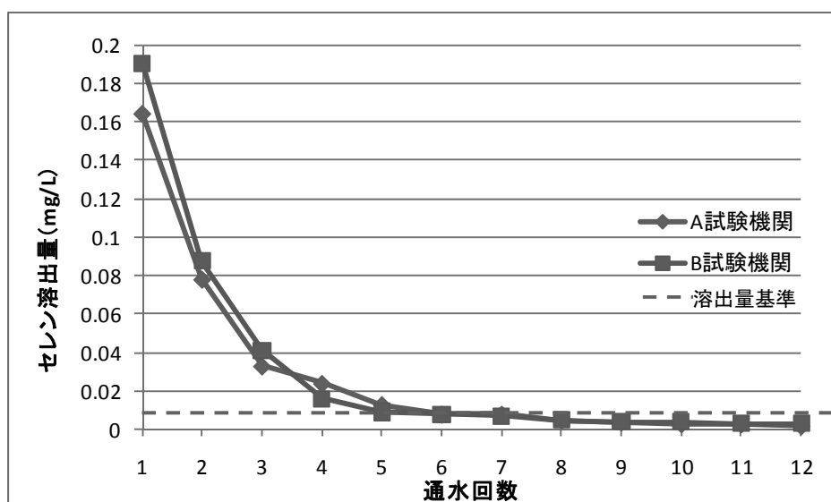
図 4 通水回数とセレン溶出量の関係
