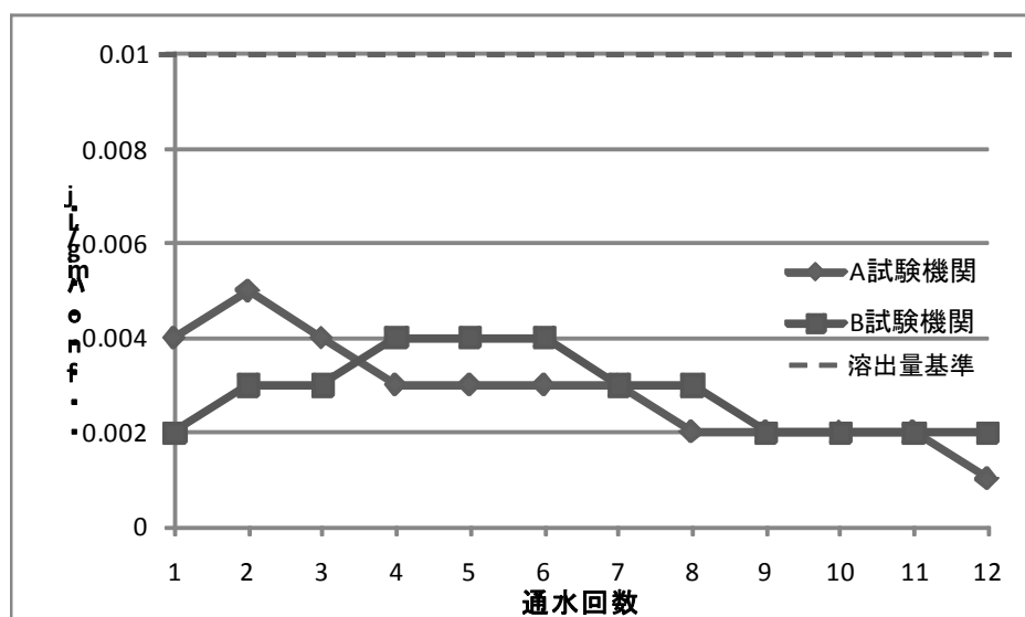
図 3 通水回数と砒素溶出量の関係
