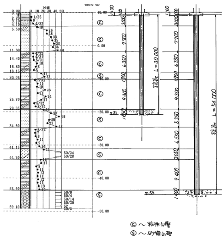
図1 建築物基礎の杭基礎設置と土質区分
