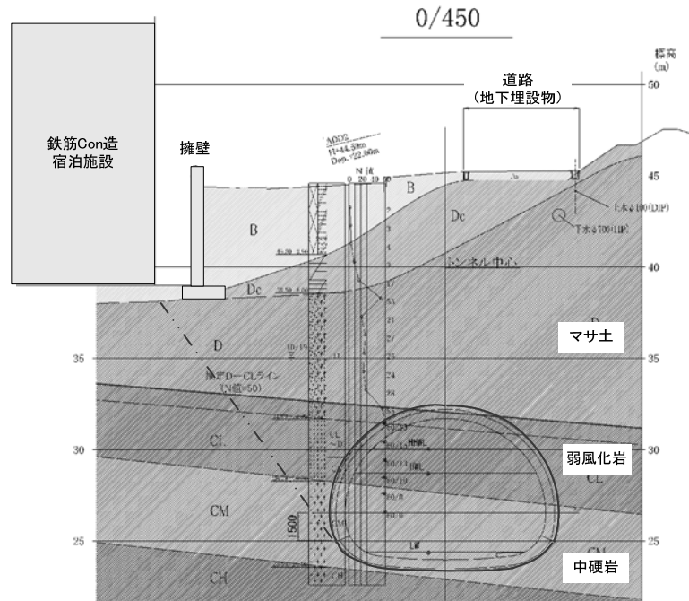
図6 硬岩混在区間の横断面図例
