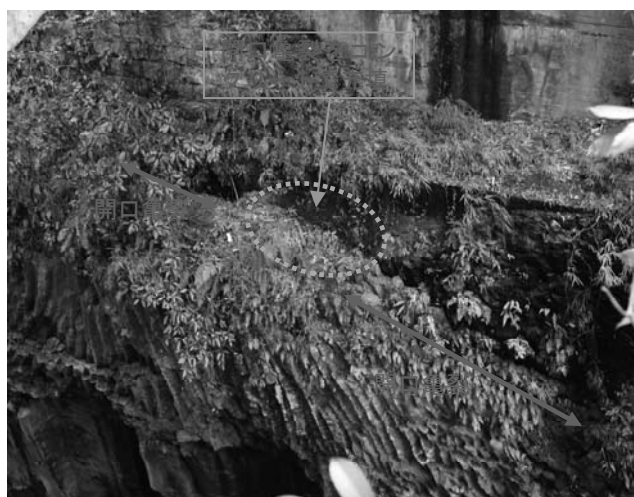
図-3 御橋橋台付近の開口亀裂
