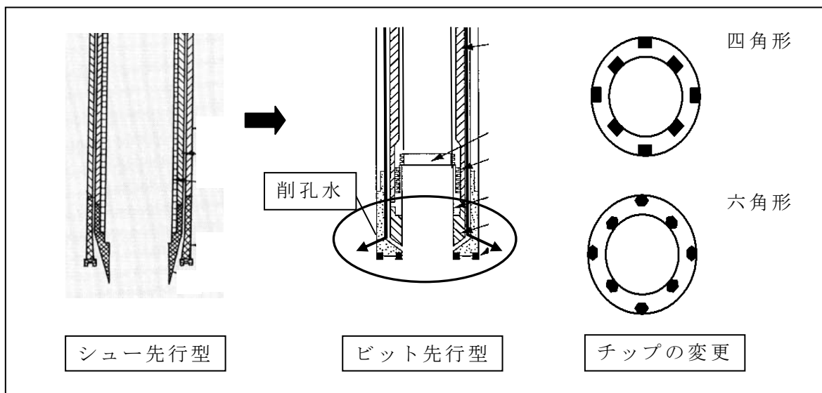
図-5 サンプラー構造及びビット 参考文献3)
