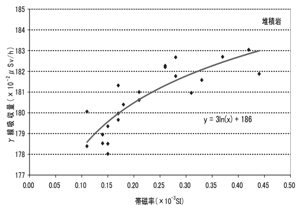
図 2 帯磁率を指標とした \gamma 線減弱実験結果
