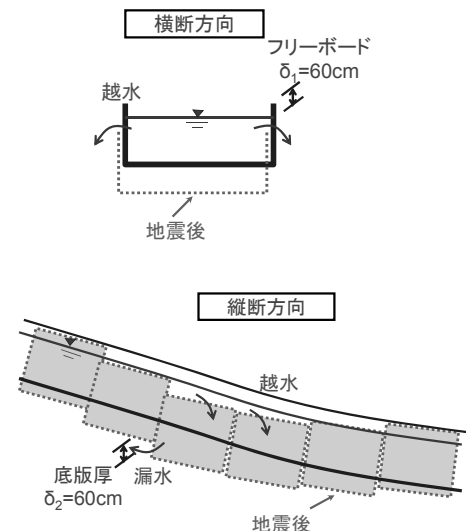
図-3 当該水路のリスク事象(限界状態)
