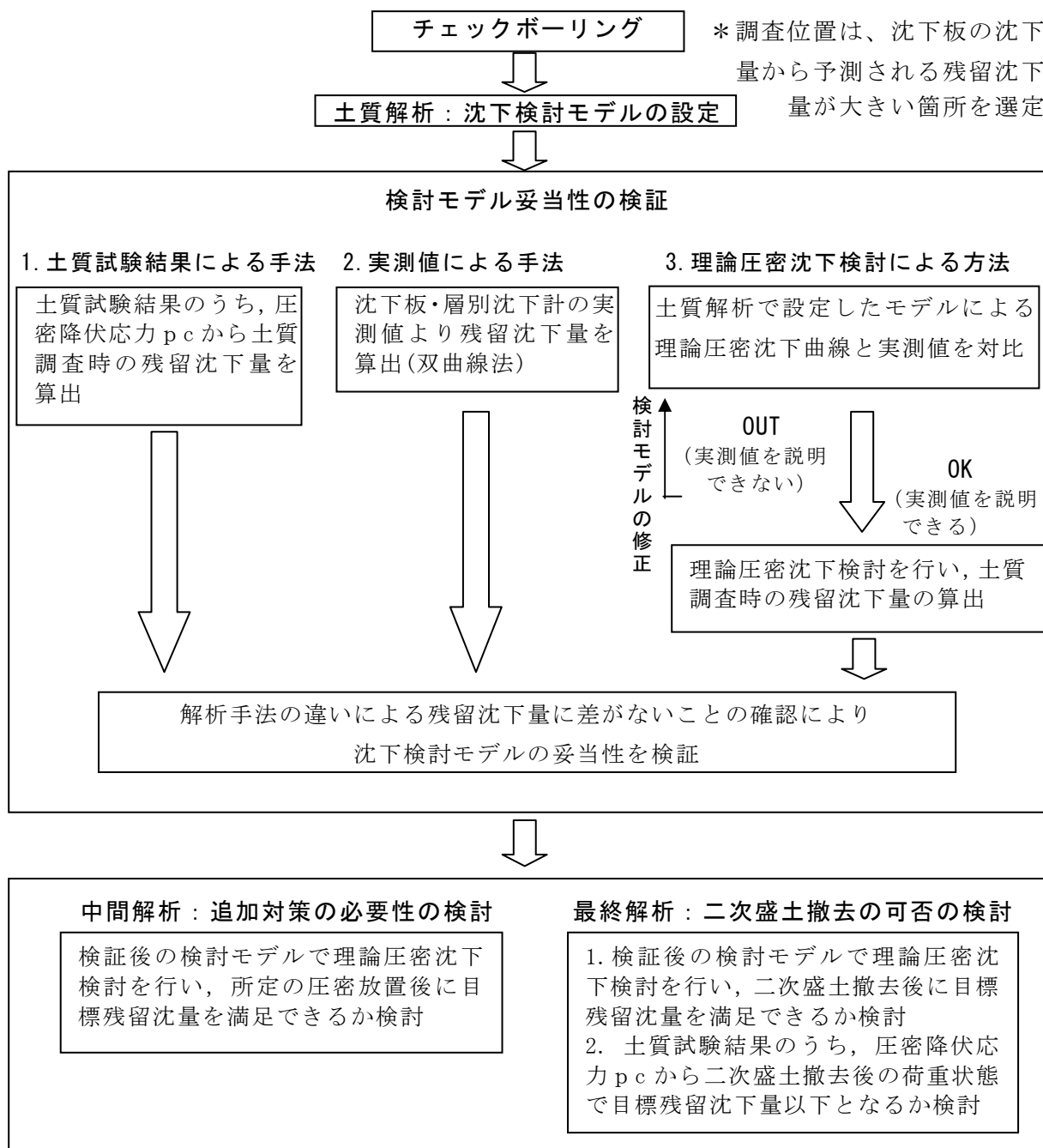
図3 沈下解析項目と検討フロー
