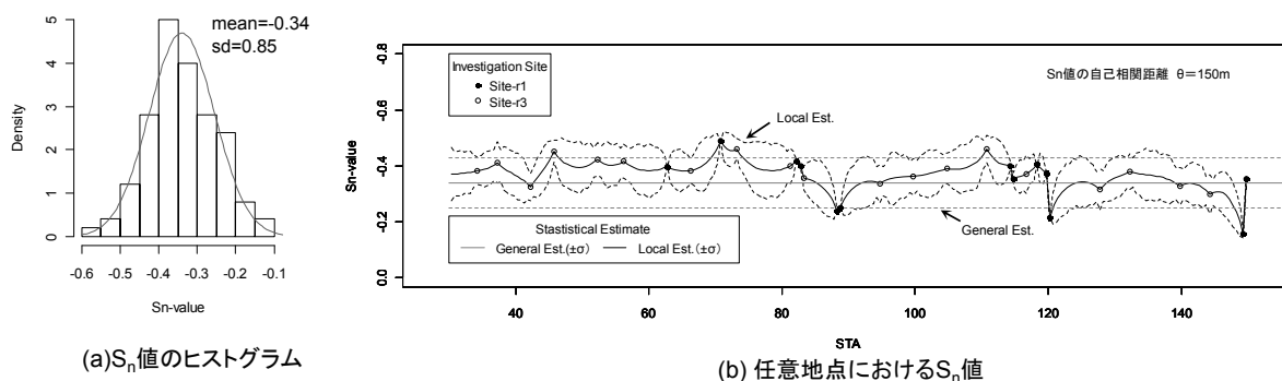
図-7 任意地点の S_n 値不確実性 (地質リスク) の定量化結果
