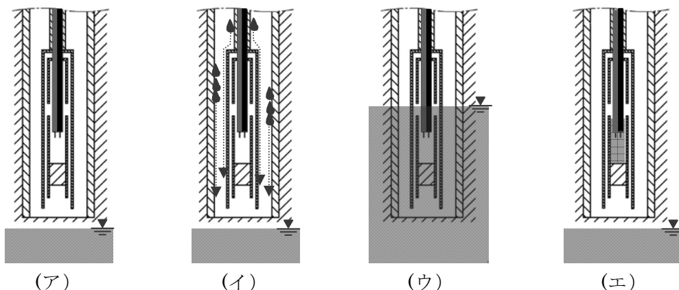
図6 センサーの構造
