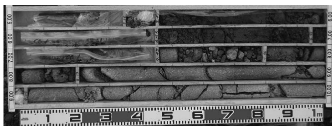
写真 3 CB.1 コア写真 (段丘堆積物～流紋岩)
