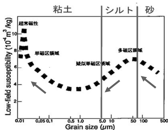
図 1 純粋なマグネタイトの単位質量当たり帯磁率（縦軸）と粒径（横軸）との関係 1)
