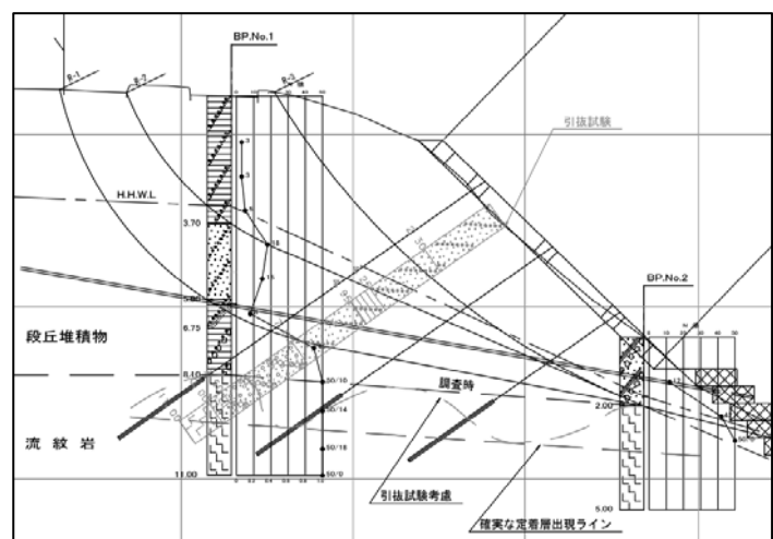
図6 模式推定断面図
