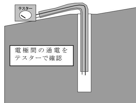
図5 地下水検知の概要
