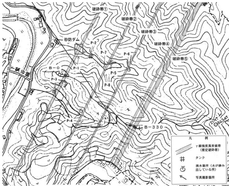
図 6 破裂帯分布と湧水地点の対応
