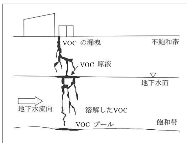
図3 VOCの浸透挙動模式図
