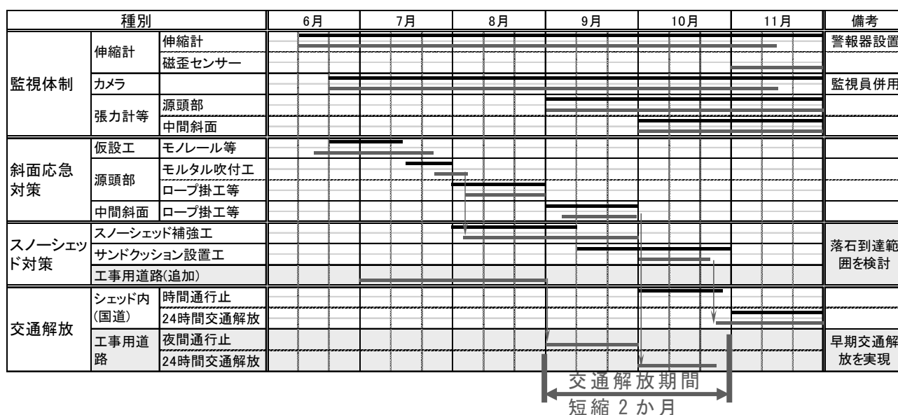
図 6 実施工程表(黒線：計画、赤線：実施)
