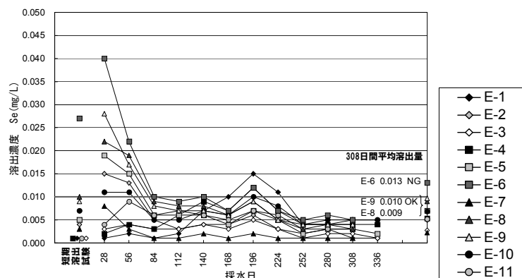
図 4 曝露試験におけるセレンの溶出濃度
