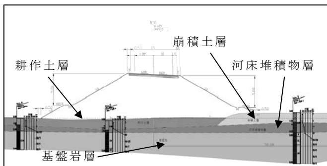
図-6 地質断面図
