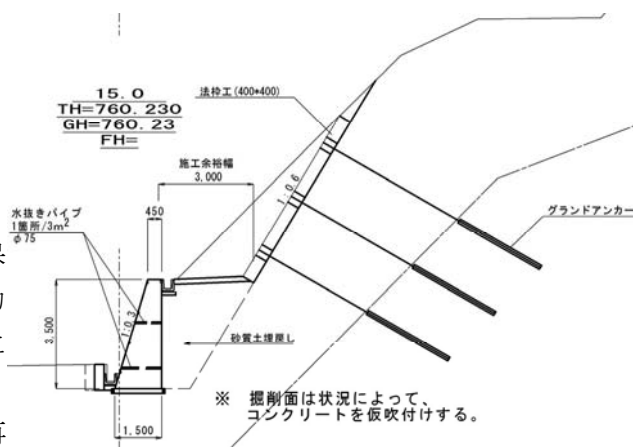
図 2.1 リスク対応方針 1（設計原案）の概要図
