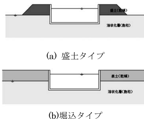
図-1 水路の構造形式
