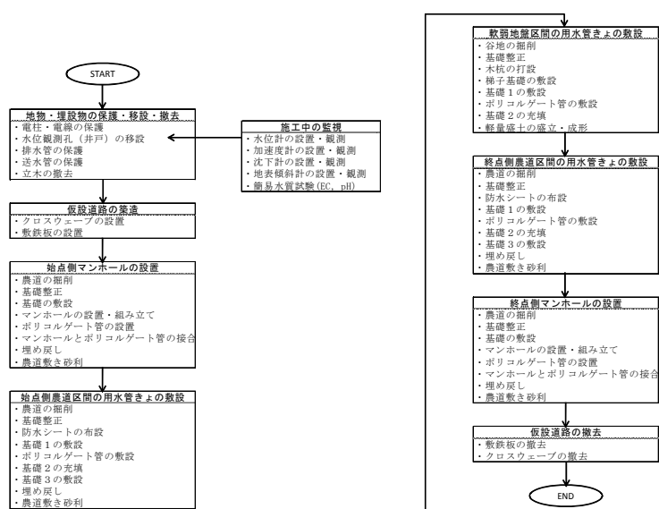
図3 施工フローの中における施工中の監視
