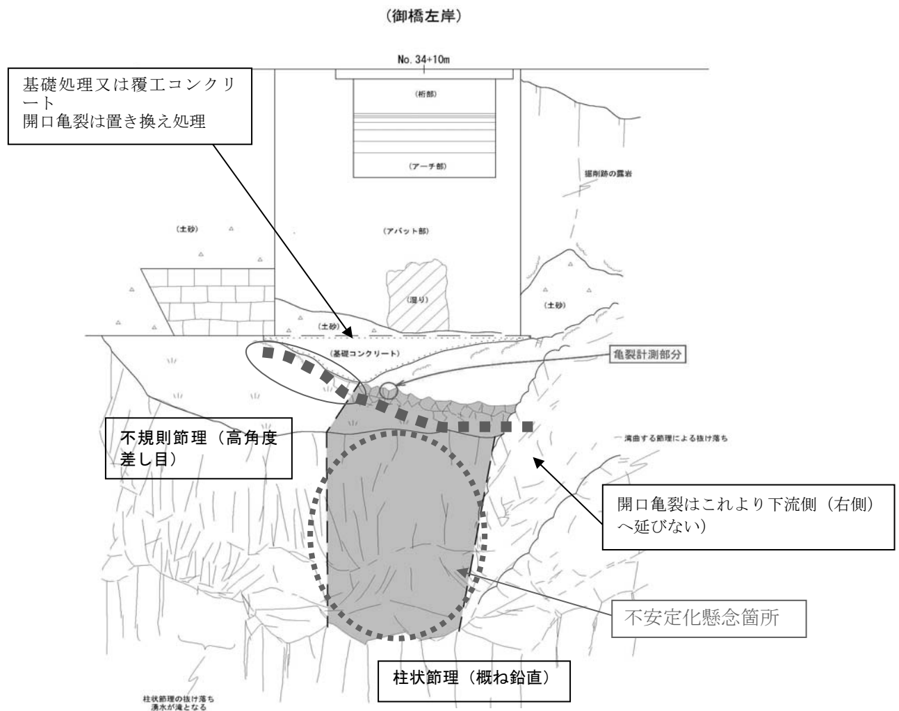
図-5 御橋左岸側の急崖部の状況（正面図）
