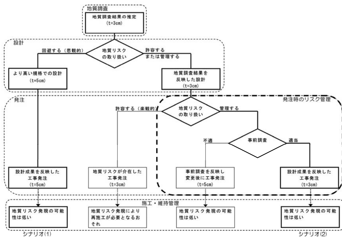
図2 事業段階と地質リスクの流れ
