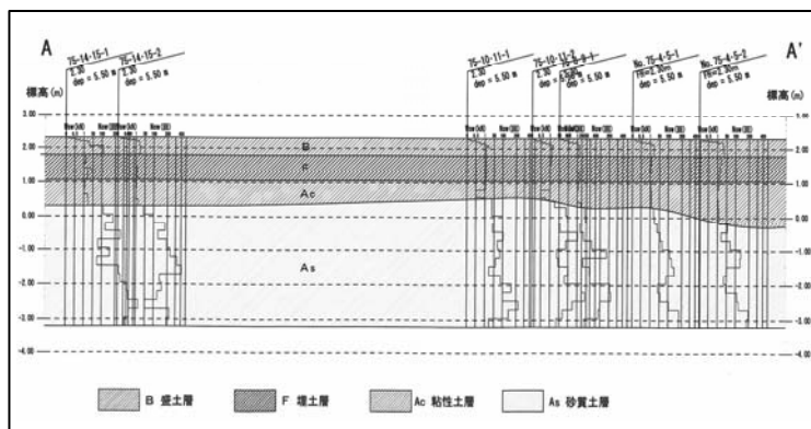
図1 地質断面図
