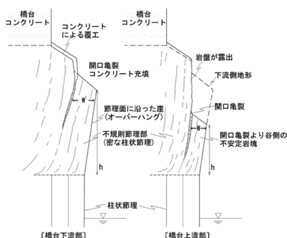
図-4 御橋橋台の模式地質断面
