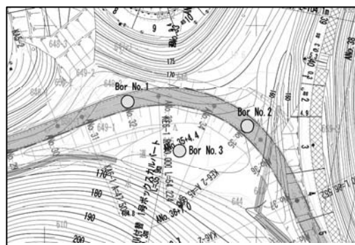
図-4 調査位置図
