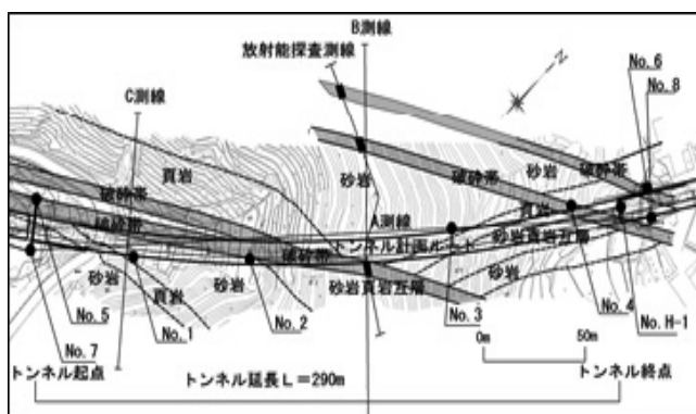
図 3 地質平面図（破砕帯分布図）
