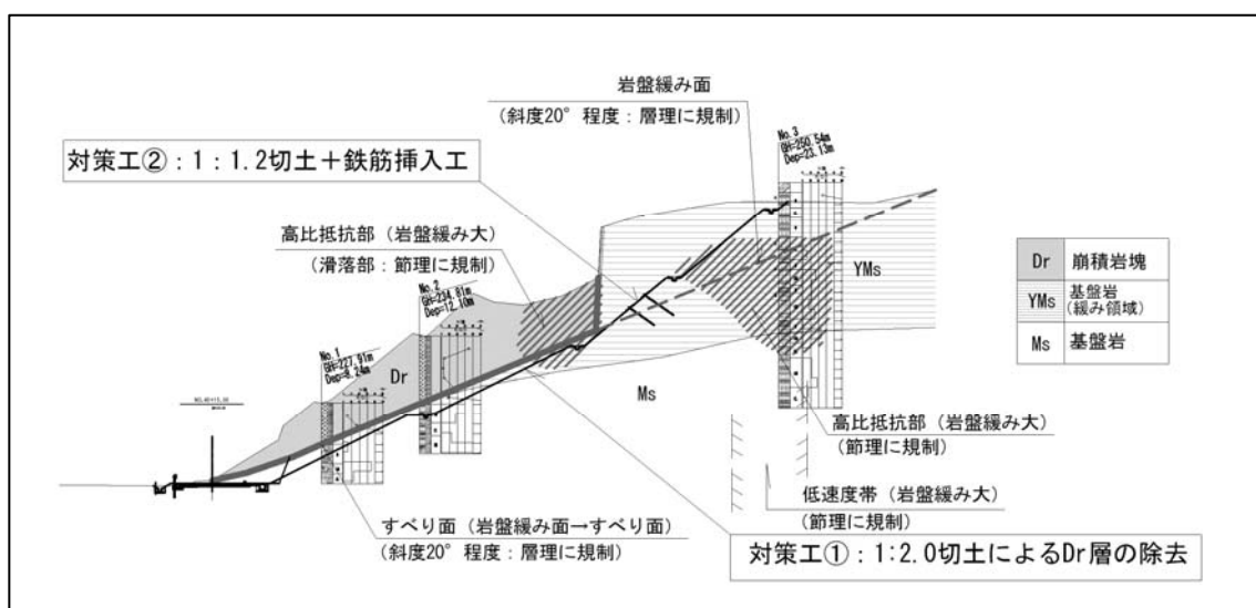
図5 調査結果と対策工の概要 (S=1/800)
