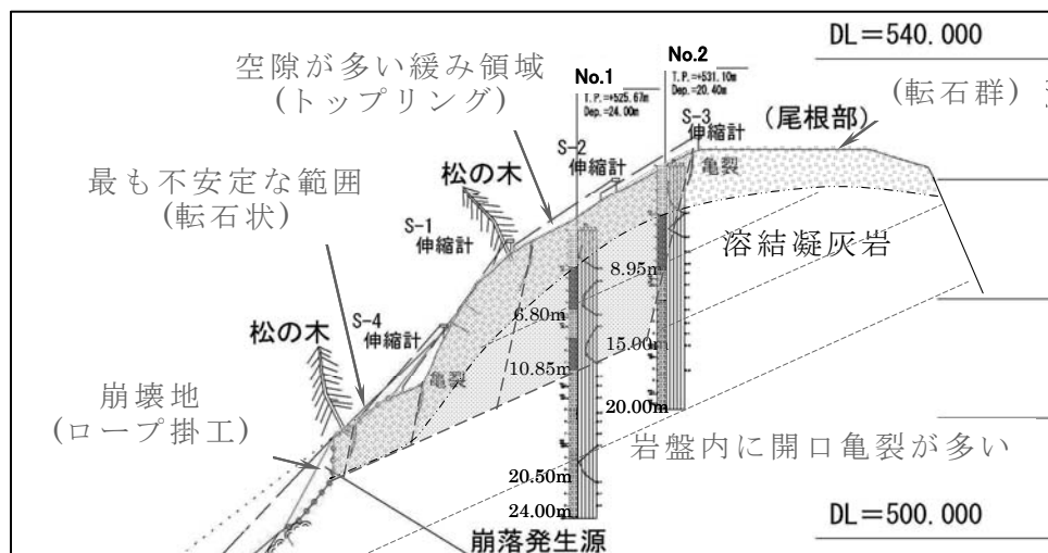
図 3 崩壊箇所背後斜面の断面
