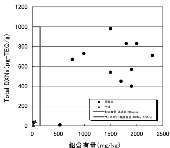
図 2 ダイオキシン類濃度及び鉛含有量との相関性
