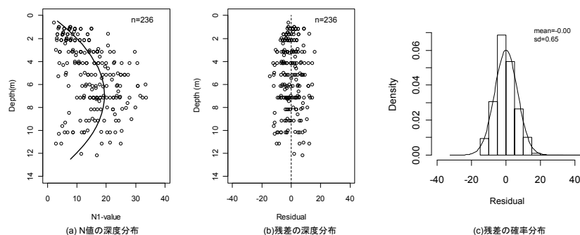
図-6 空間的バラツキのモデル化と S_n 値の推定結果
