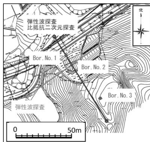
図4 調査地点位置図
