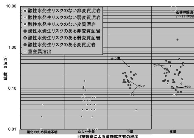
図 1 目視観察による黄鉄鉱含有の程度と S/Ca モル比関係図
