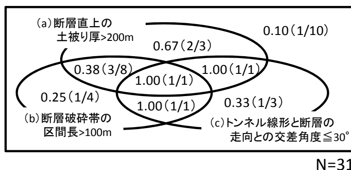
図5 地質学的素因の集合分布図
