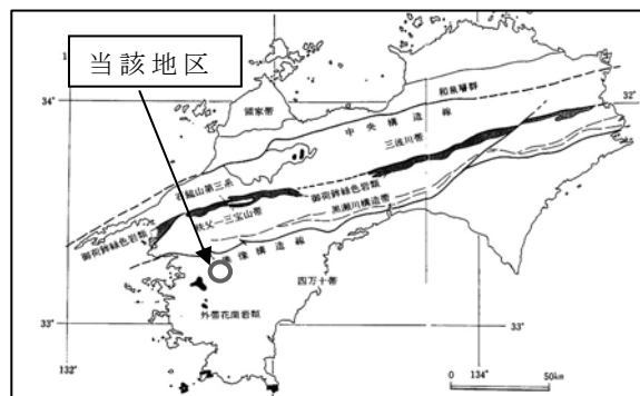
図-3 愛媛県地質図
