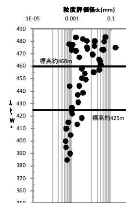
図 2 阿蘇谷湖成層の堆積構造
