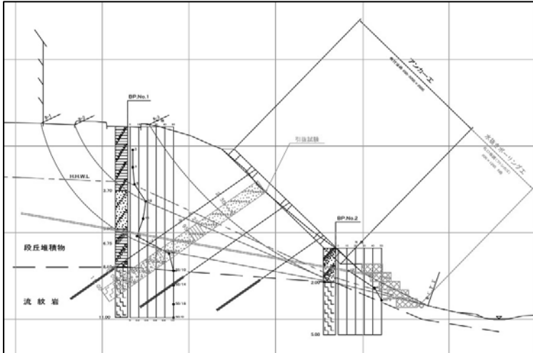
図4 対策工断面図2（引抜試験データは投影）
