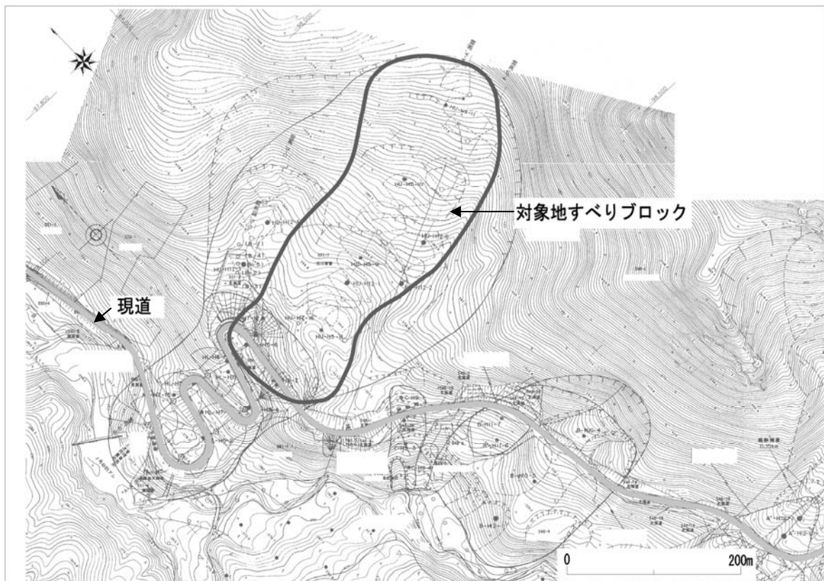
図1 現道と地すべりの関係
